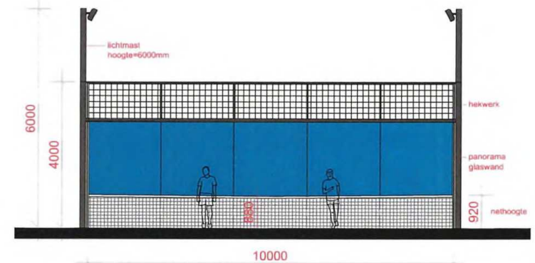
DOORSNEDE B-B
