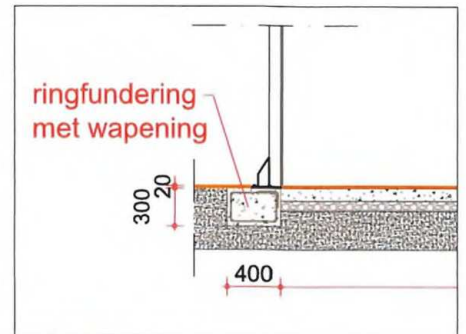
detail schaal 1:20
