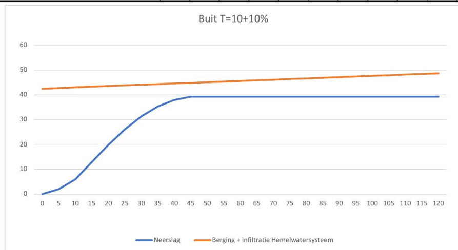
Grafiek Bui T=10+10%
