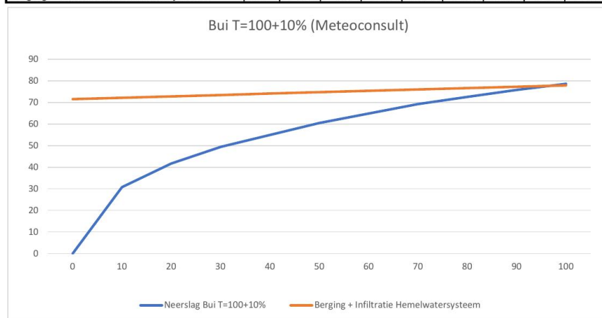
Grafiek Bui T=100+10%
