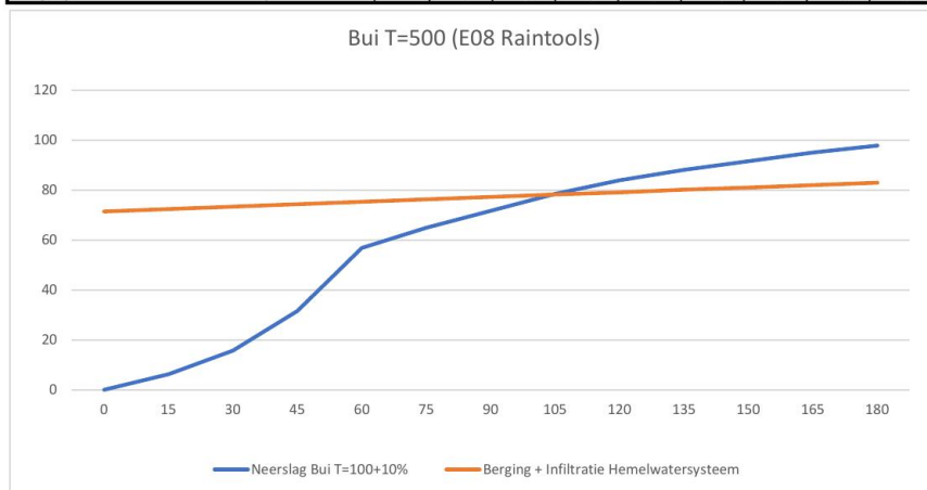
Grafiek Bui T=500 (E08 Raintools)
