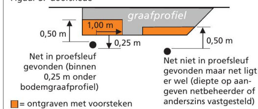
Figuur 3: doorsnede
