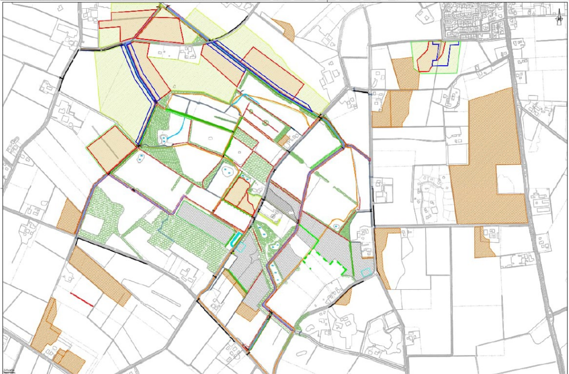
Figuur 2: Inrichtingen plan met te nemen maatregelen.
