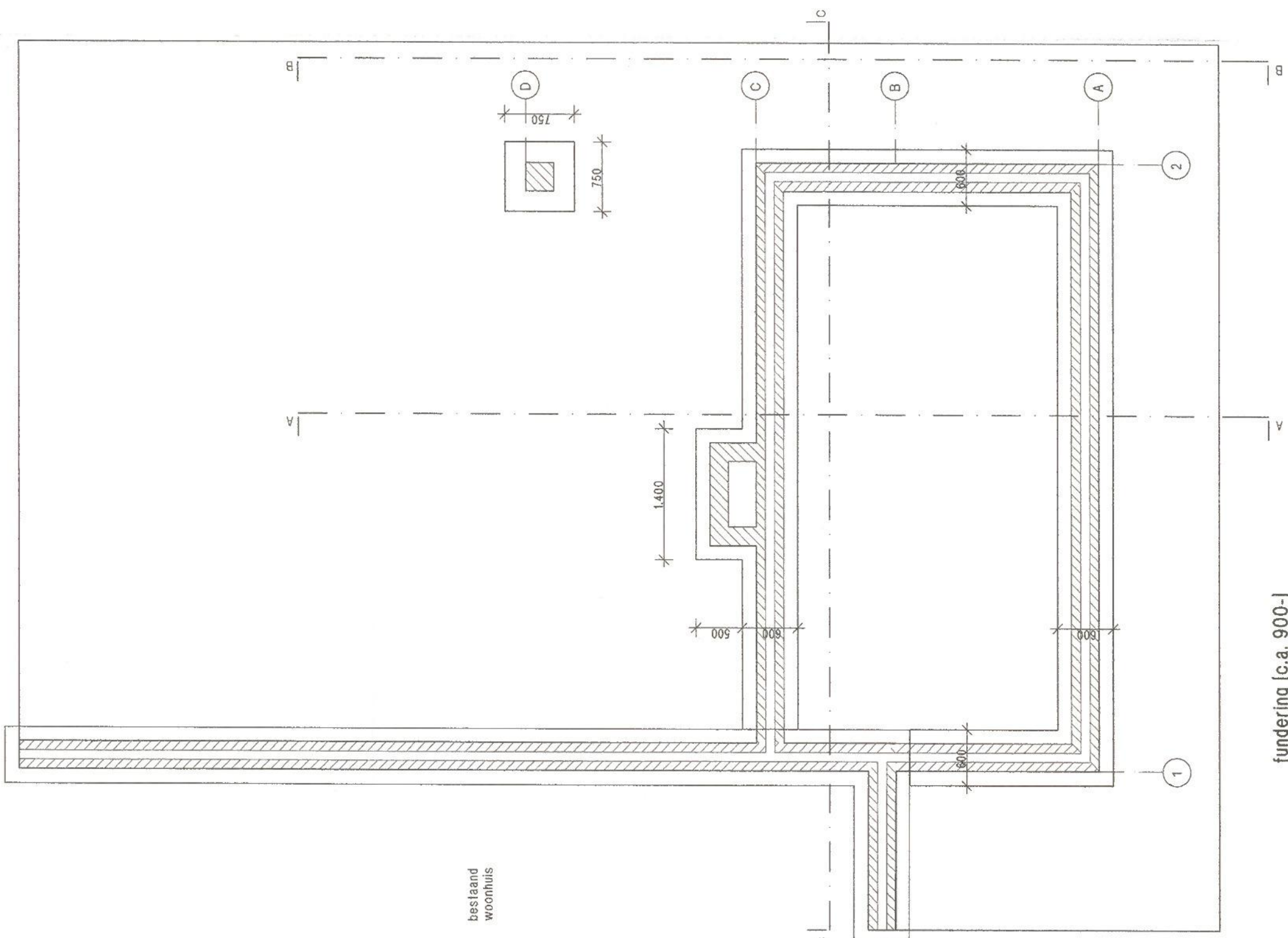
begane grondvloer (peil)
