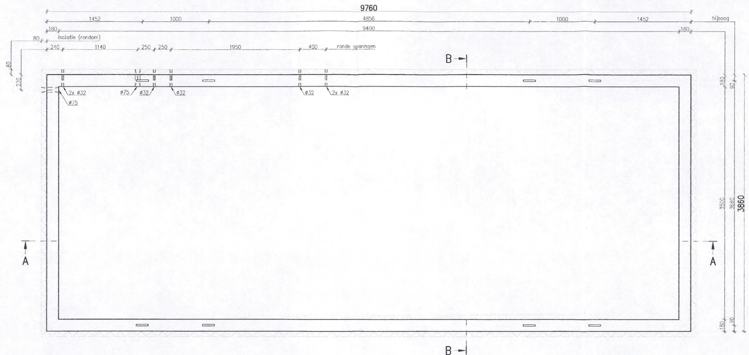
bovenaanzicht stortzijde
