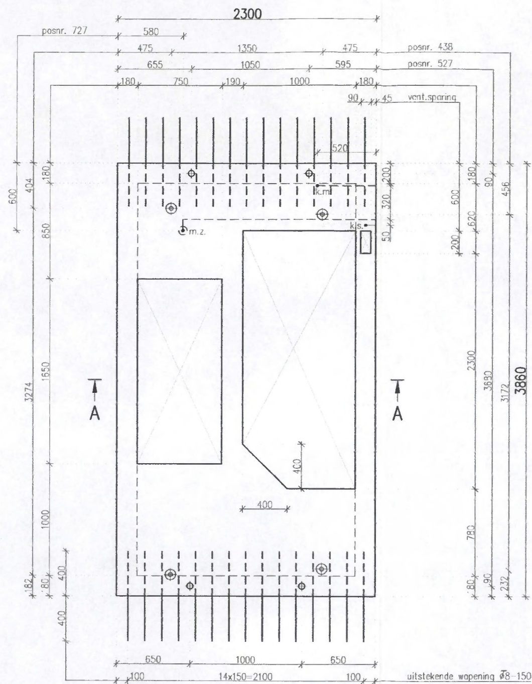
kelderdek stortzijde
