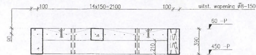
doorsnede A-A
