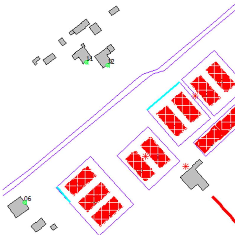
Figuur 6 Noodzakelijke geluidschermen om in de toekomstige situatie te kunnen voldoen aan de grenswaarden/maatwerkvoorschriften (situatie padelbanen 3 uur in gebruik)
