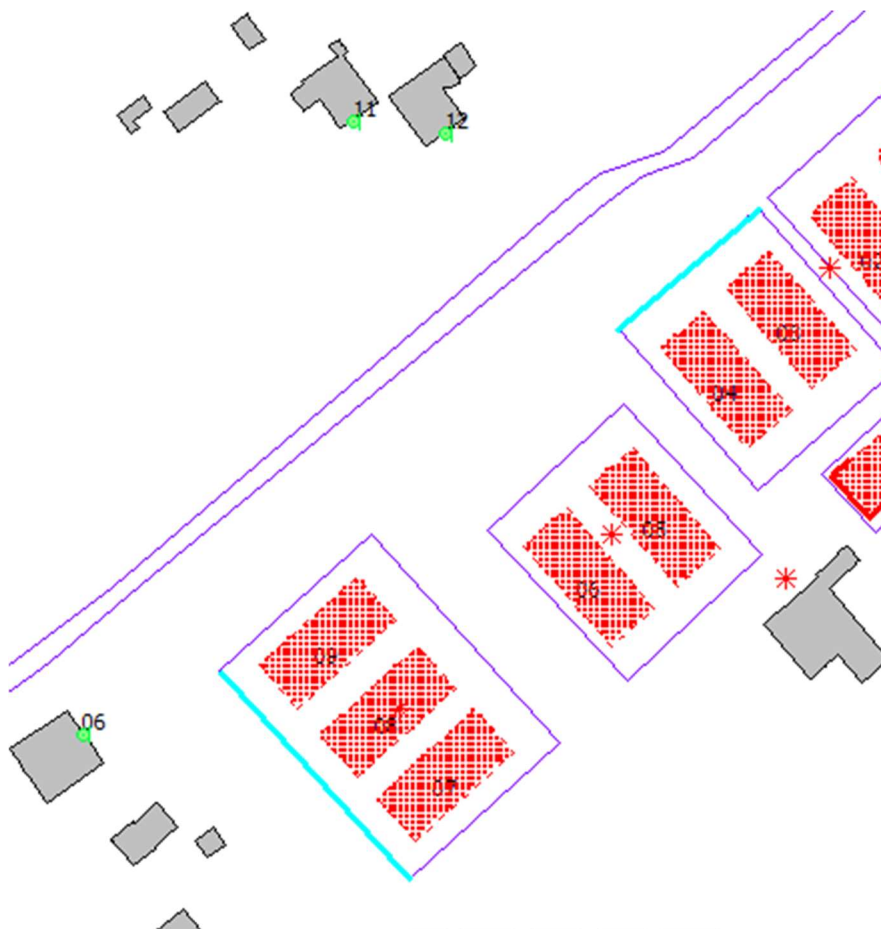
Figuur 7 Noodzakelijke geluidschermen om in de toekomstige situatie te kunnen voldoen aan de grenswaarden/maatwerkvoorschriften (situatie padelbanen 4 uur in gebruik)
