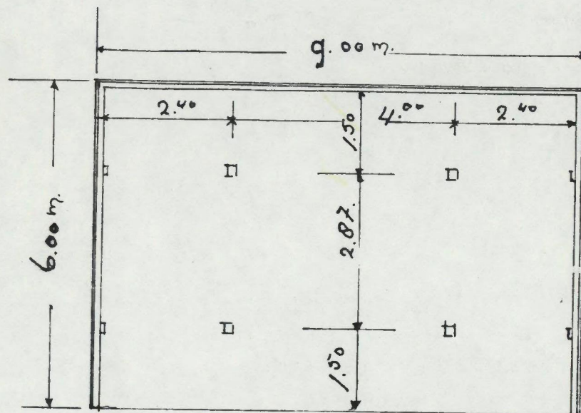
~ platte-grond ~
