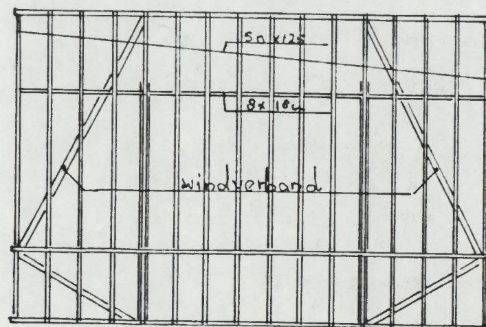
~ kap-plan ~
