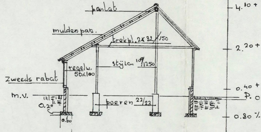
~ doorsnede ~
