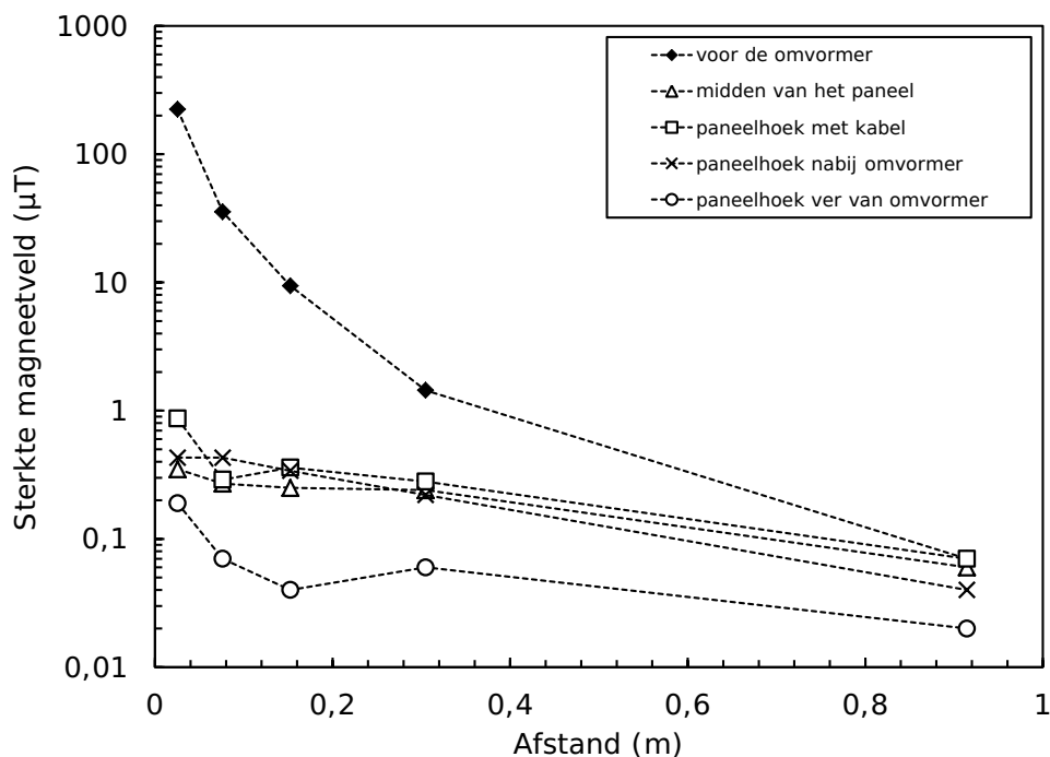
Figuur 3. Gemeten sterkten van het magnetveld op diverse afstanden van een paneel waarop de omvormer aan de achterkant is gemonteerd (Bron: 5.1.2e, 1997)
