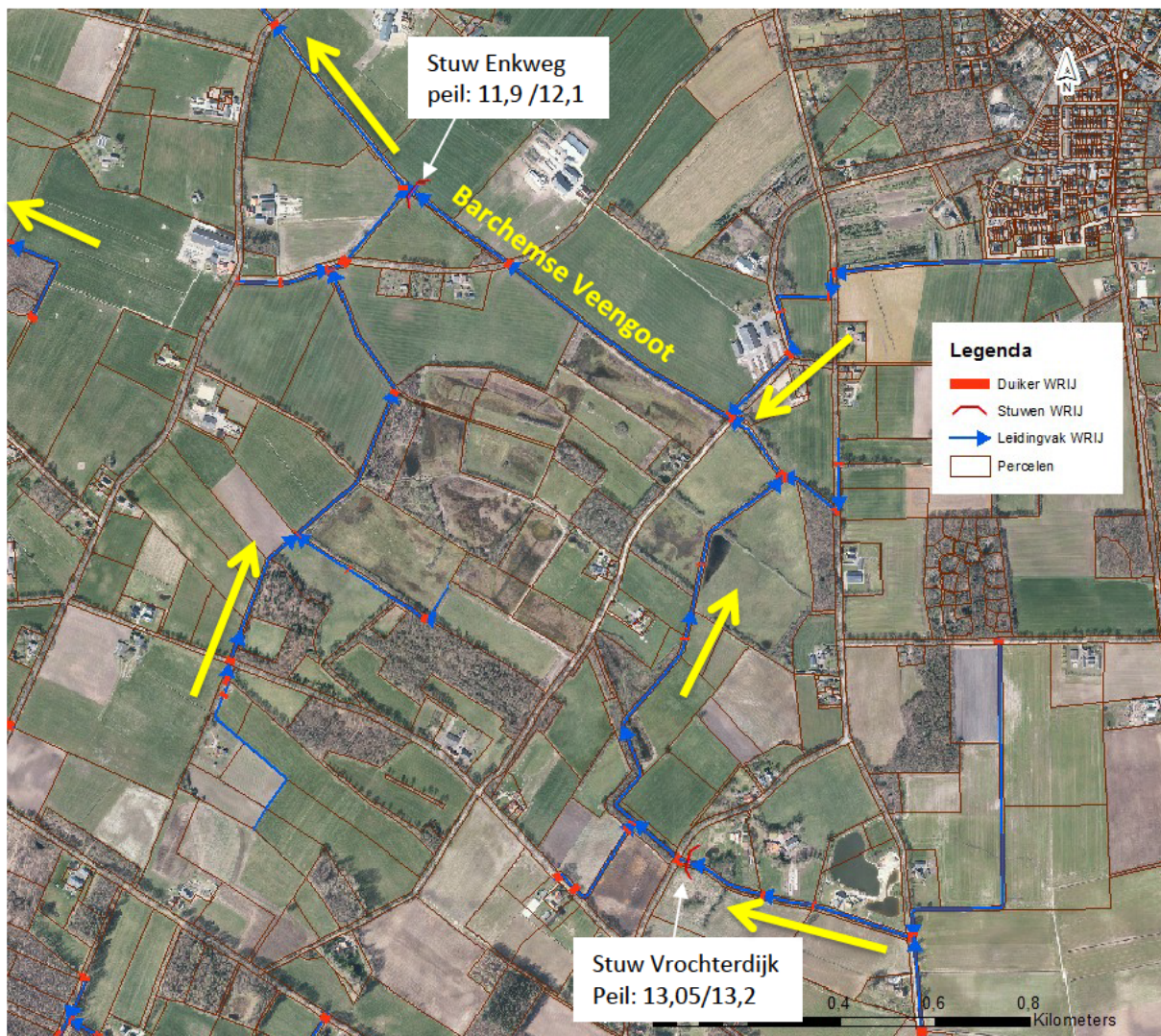
Figuur 4: Afwateringsrichting.
