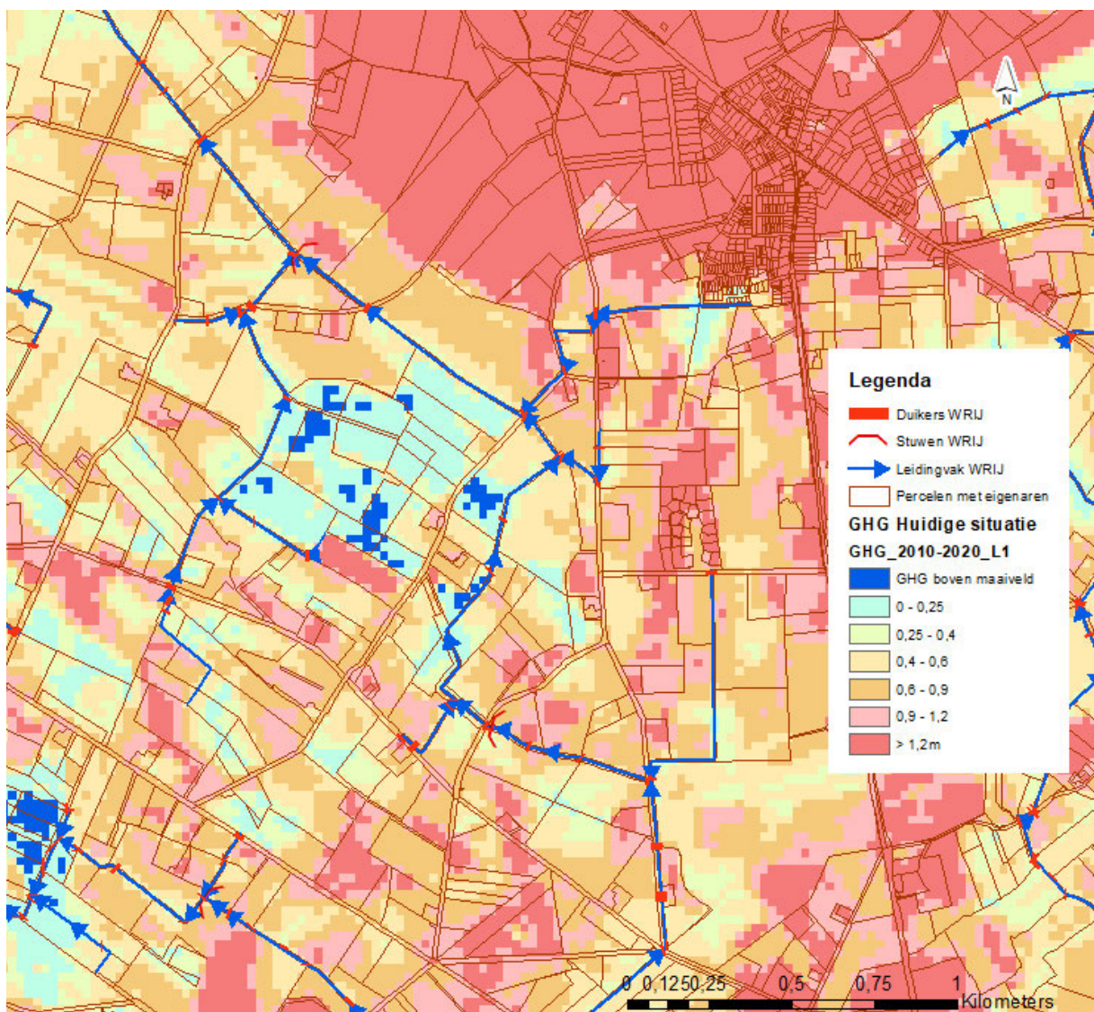
Figuur 5: Actuele Gemiddeld Hoogste Grondwaterstand (GHG) volgens het grondwatermodel AMIGO als gebruikt voor de effectenstudie. In kleur is de GHG in cm min maaiveld te zien.
