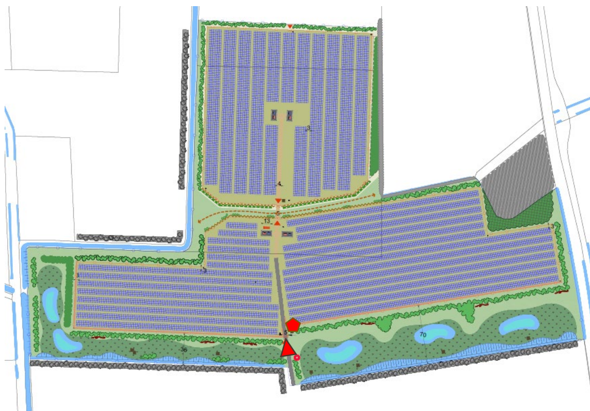
Figuur 4: Inrichtingstekening Zonnepark en Ecologische Verbindingszone (zie ook Bijlage 1)
