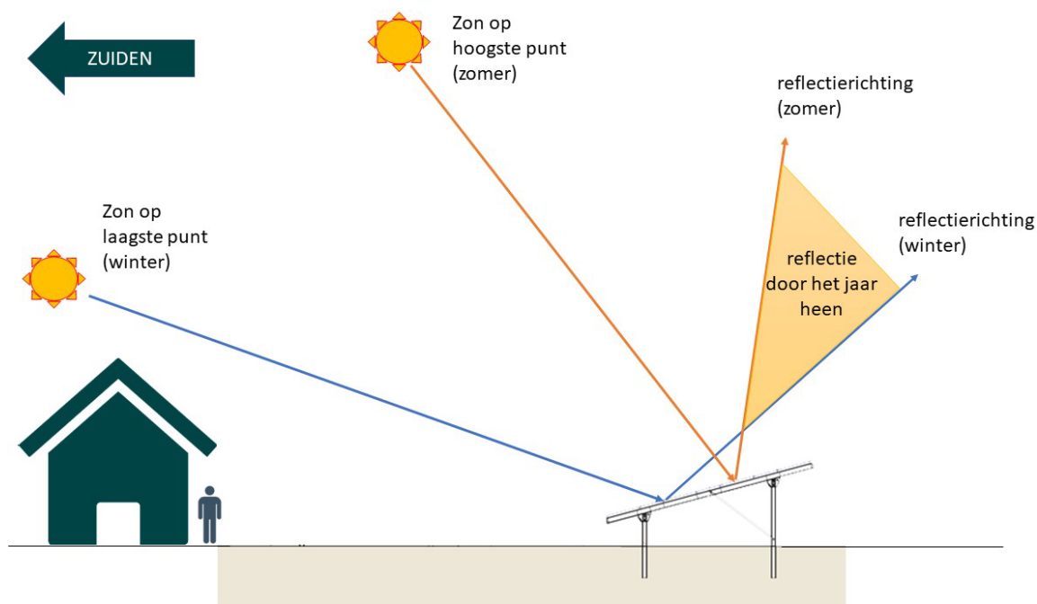
Figuur 17: Weerkaatsing bij een zuidopstelling
