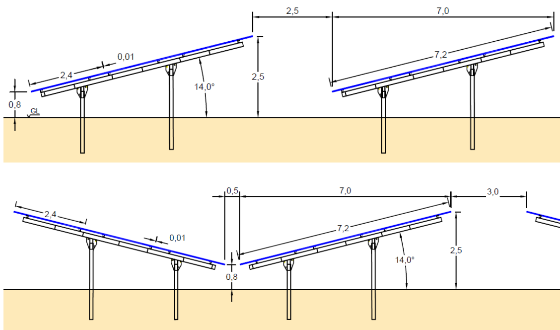
Figuur 6: principetekening beoogde constructies: boven de zuidopstelling, onder de oost/westopstelling in 'vlindervorm'.
