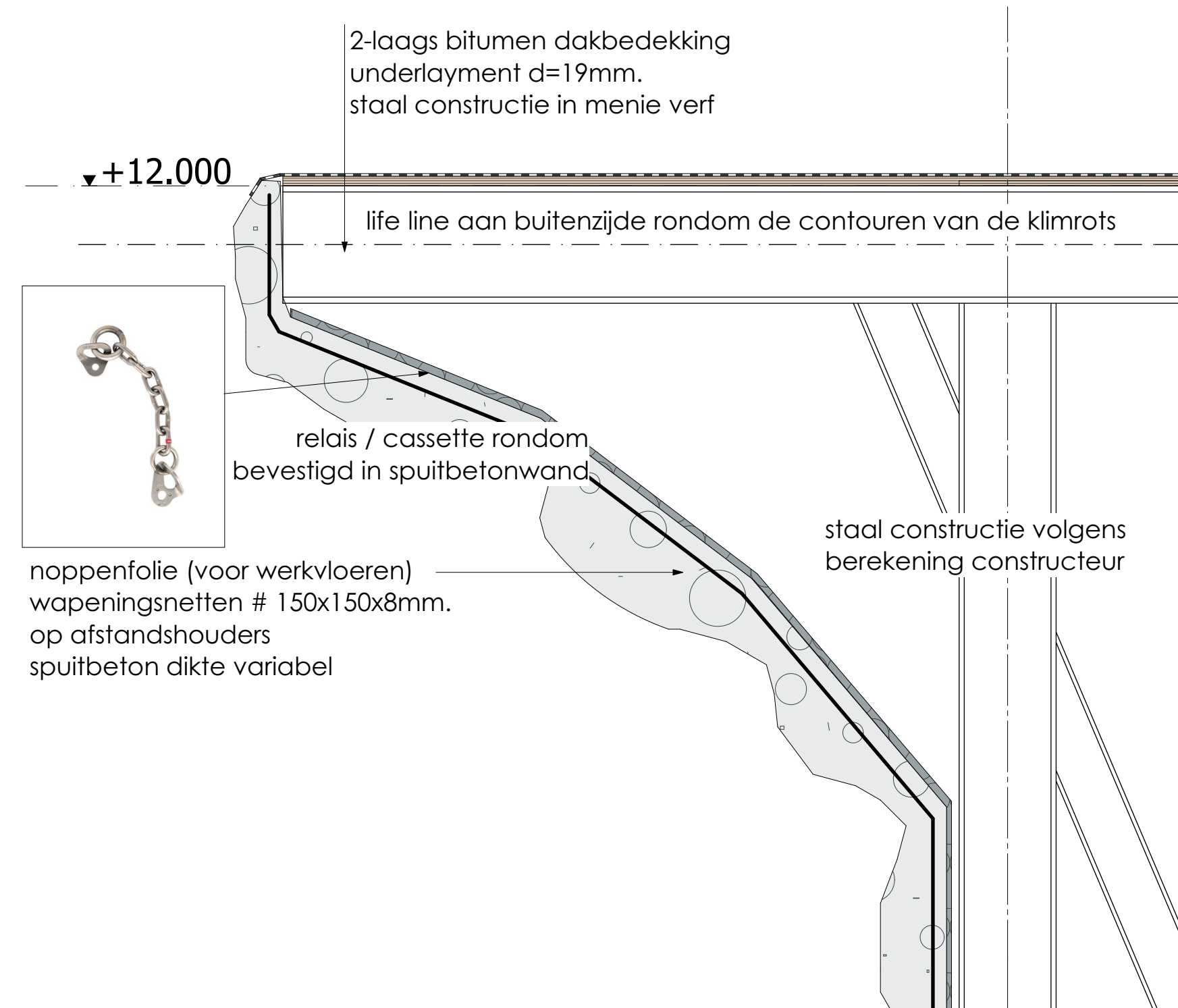
PRINCIPE DOORSNEDE D-D
