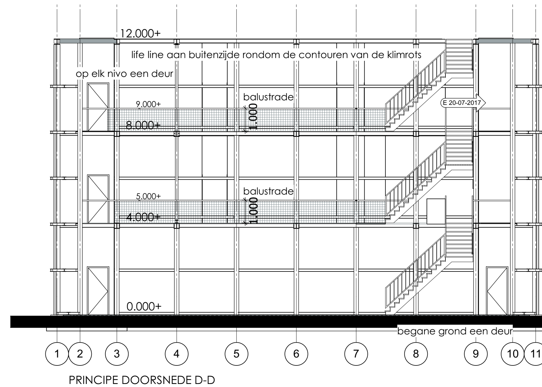
PRINCIPE DOORSNEDE D-D
