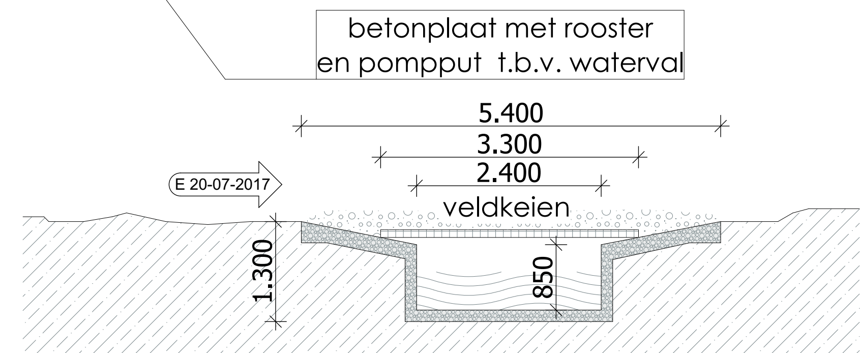
principe doorsnede 1:50
