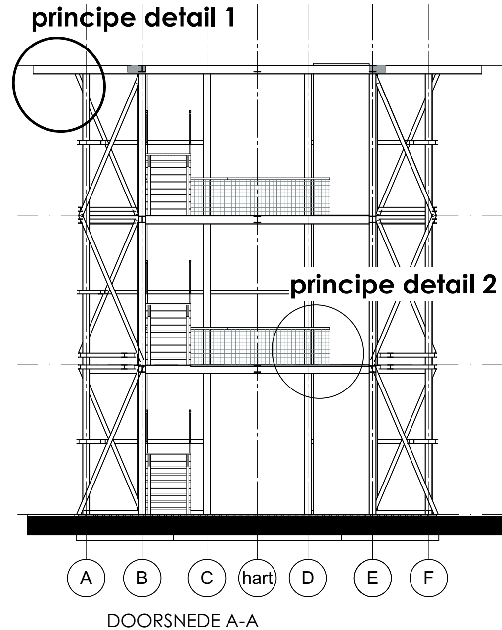
DOORSNEDE A-A
