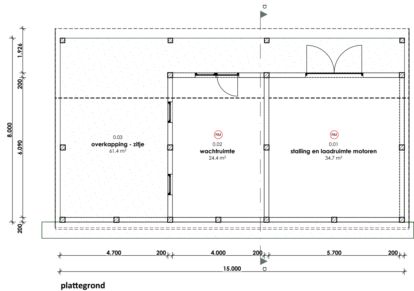
plattegrond
