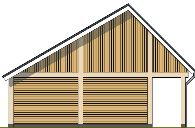
linkerzijgevel
