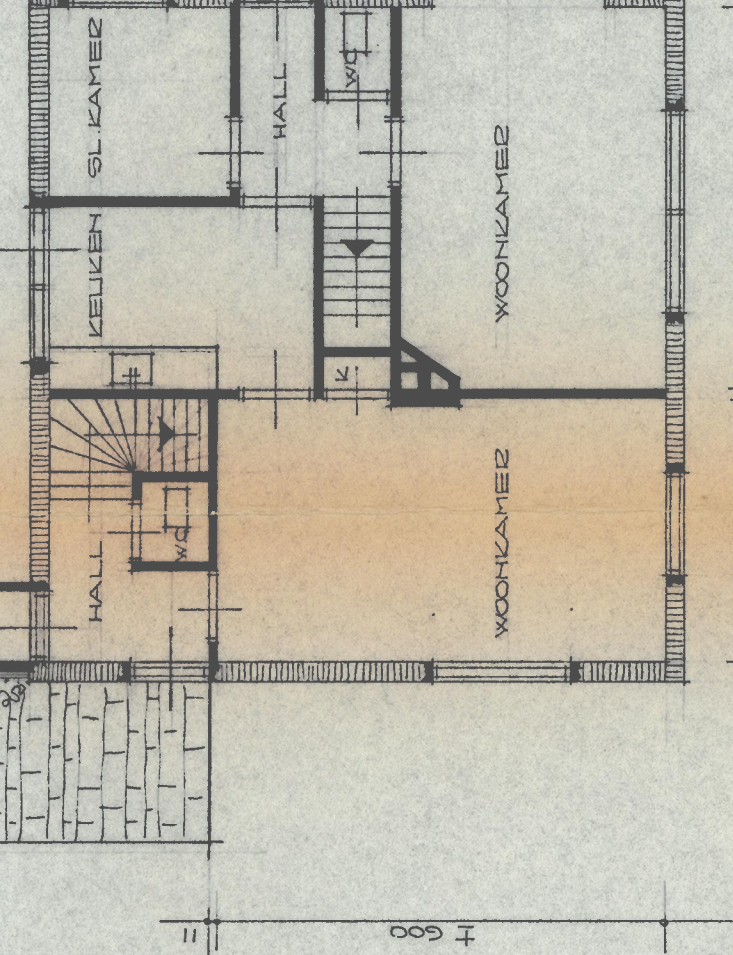
BEGANE GROND
