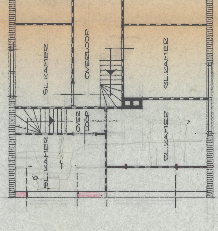
VERDIEPING
