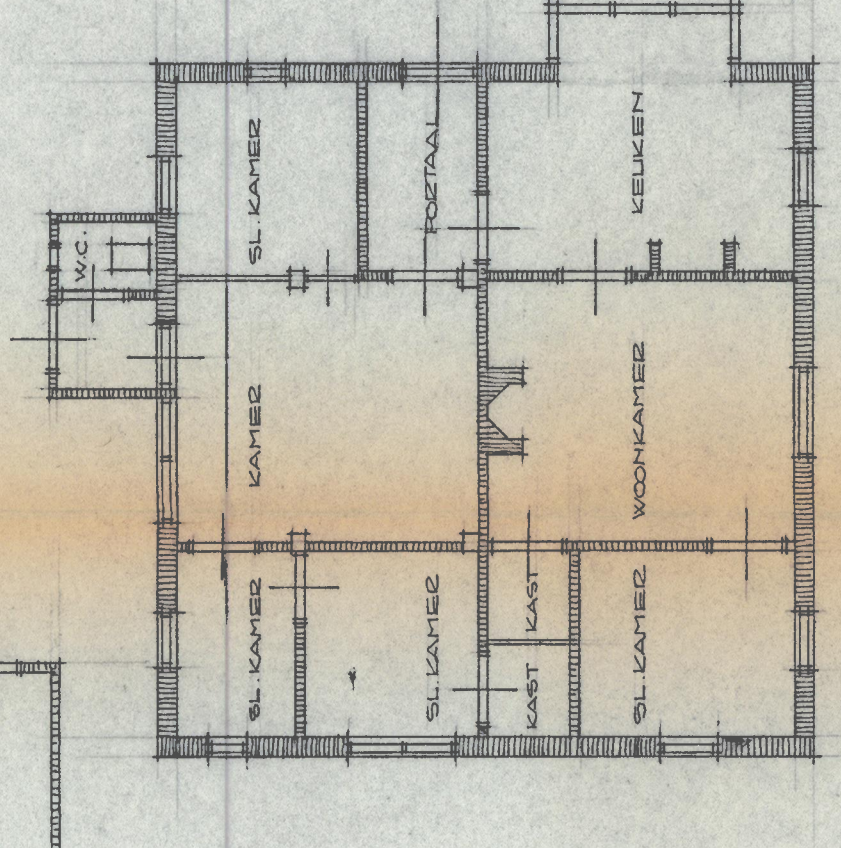
PLATTEGROND
